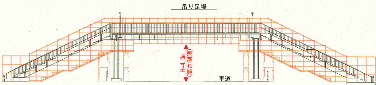
吊り足場計画図
